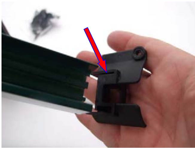
9° inserire zoccolo parte inferiore della guida
