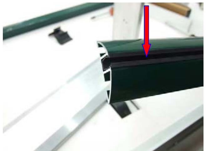
24° spessore guida FurBy mm.12
