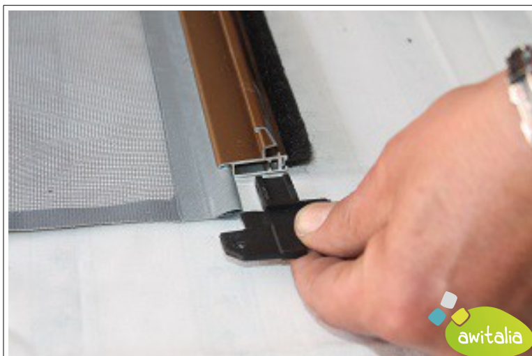
31- Inserire il corsoio laterale
