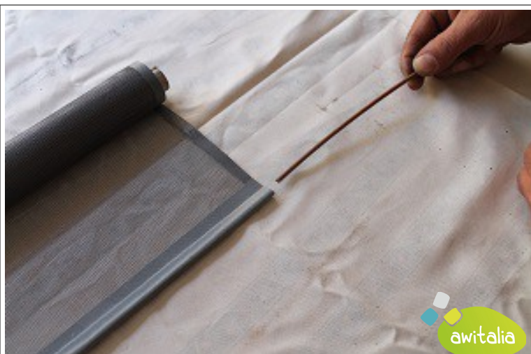
28- Infilare il tondino nella tasca/fettuccia
