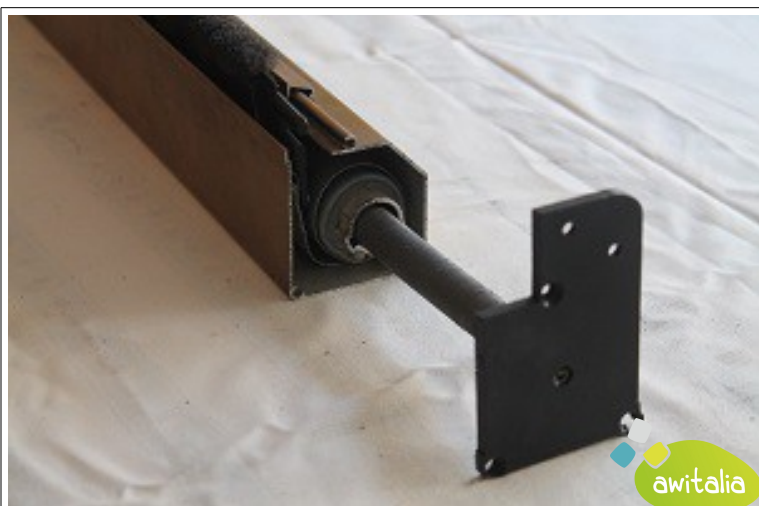
43- Inserimento del tappo con molla
