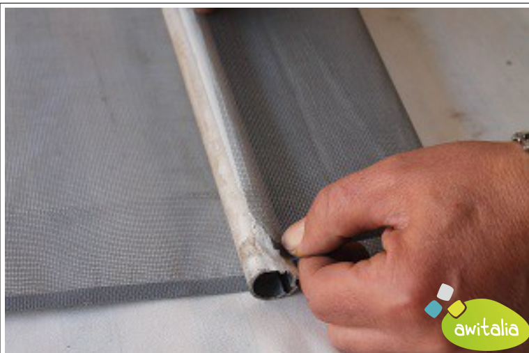
24- Attaccare la rete al rullo centrandola
