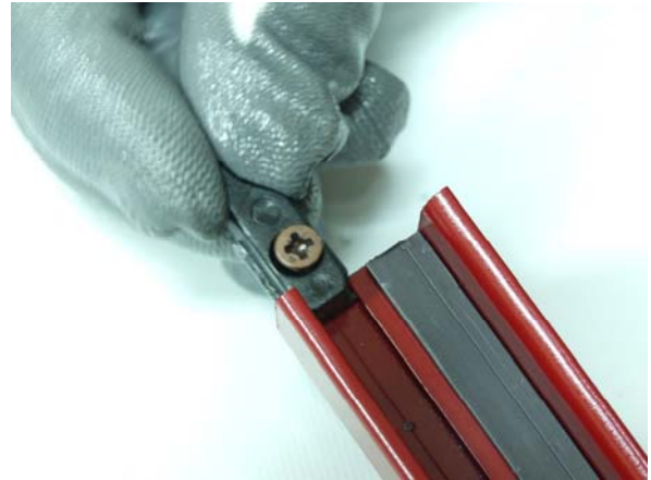
6 Inserimento fermo guida superiore ed inferiore
