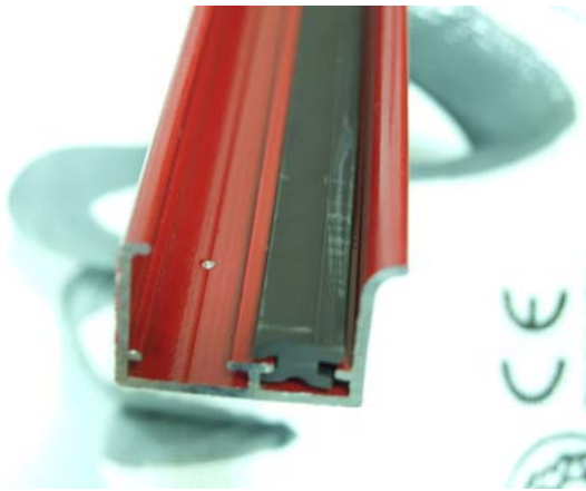
5 Guida frontale per aggancio magnetico
